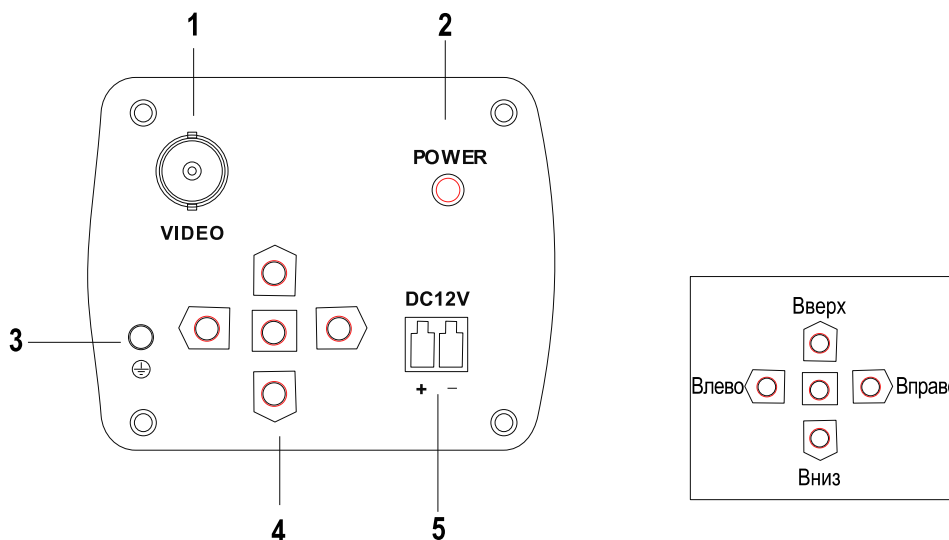
Рис. 2.2. Задняя панель
