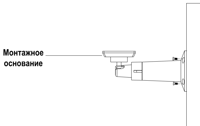
Рис. 3.2. Установка кронштейна с монтажным основанием
