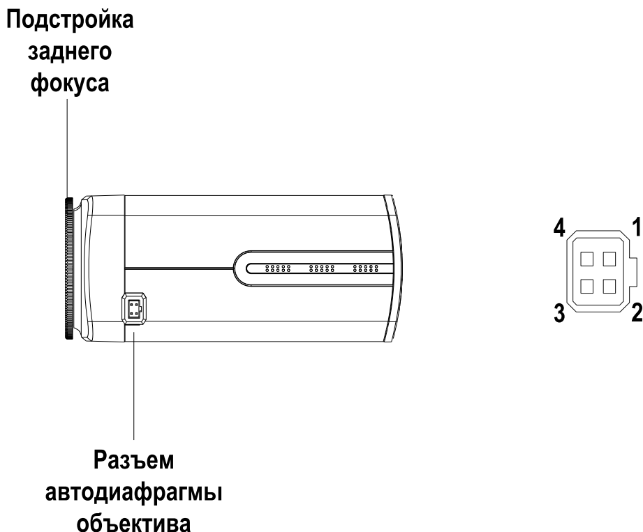
Рис. 2.1. Боковая панель
