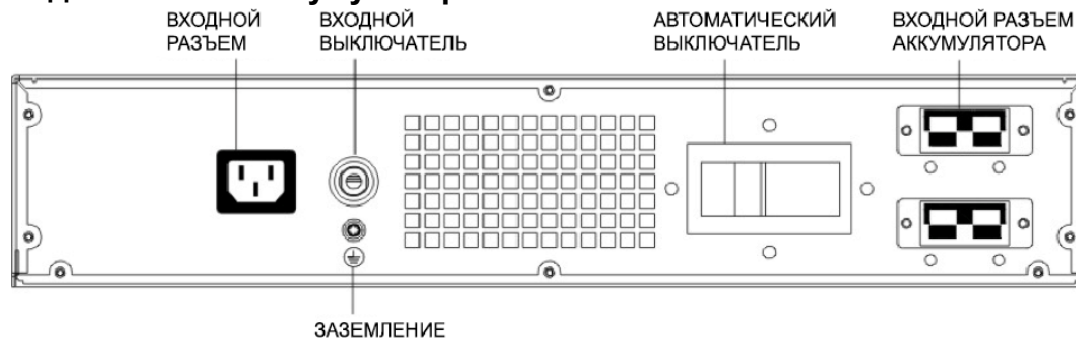
Рисунок 2 Задняя панель аккумуляторного блока 1 кВА
