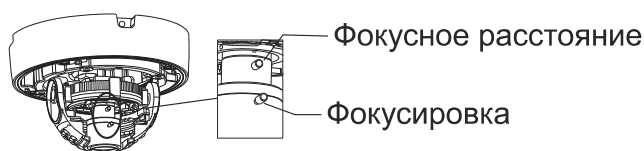
Рис. 5.6. Регулировка фокусного расстояния и фокусировки
